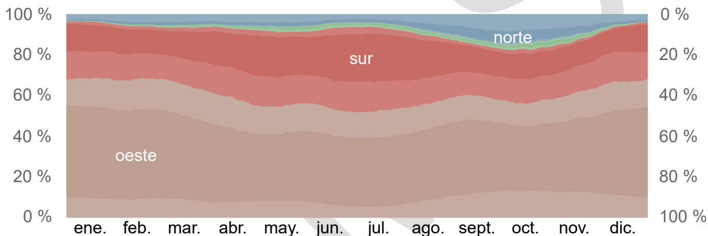
Dirección del viento en Barrancabermeja
