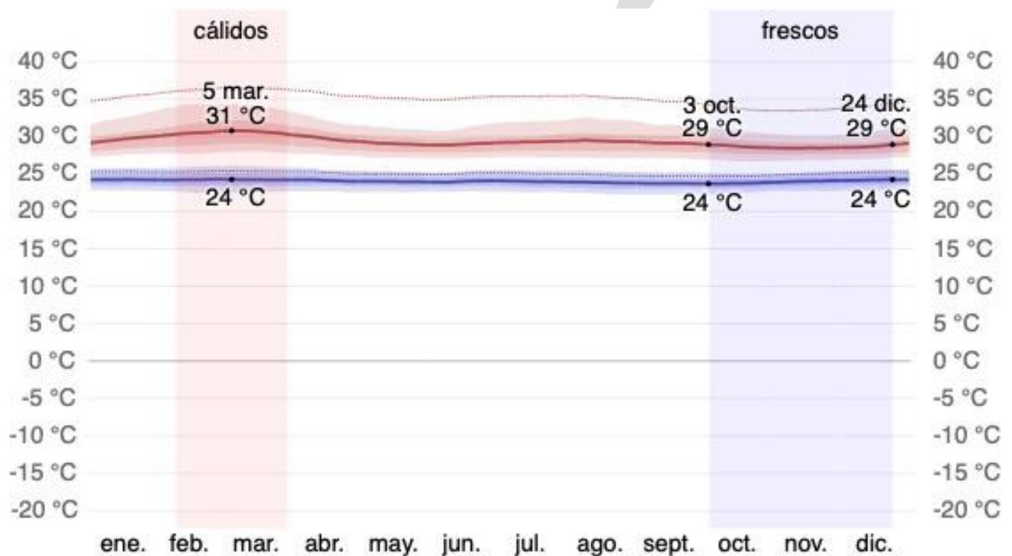
Temperatura máxima y mínima promedio en Barrancabermeja
