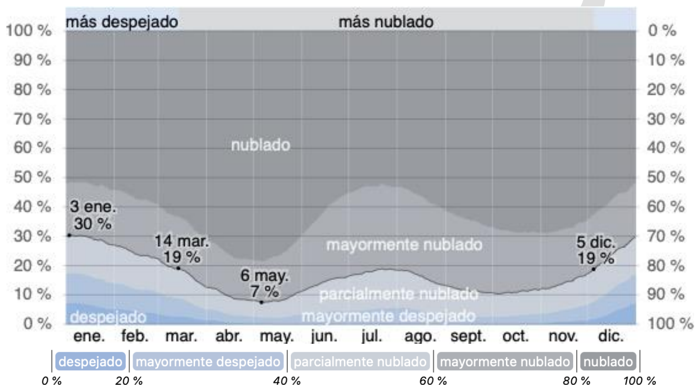
Categorías de Nubosidad en Barrancabermeja
