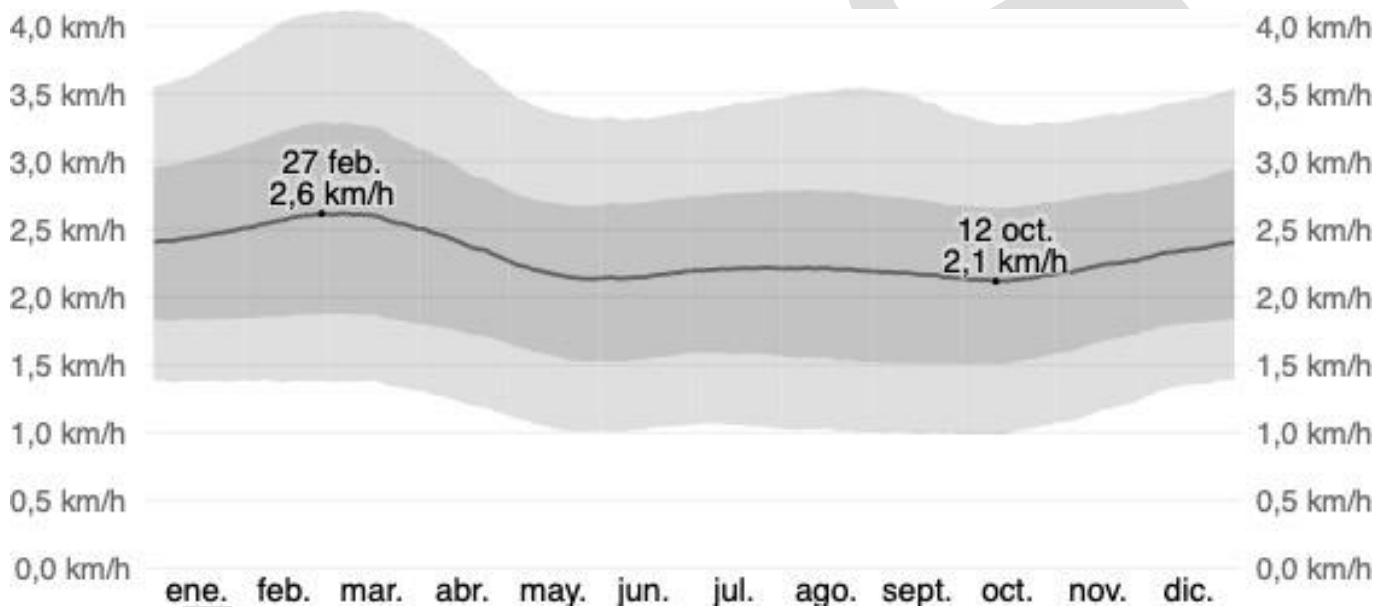
Velocidad promedio del viento en Barrancabermeja
