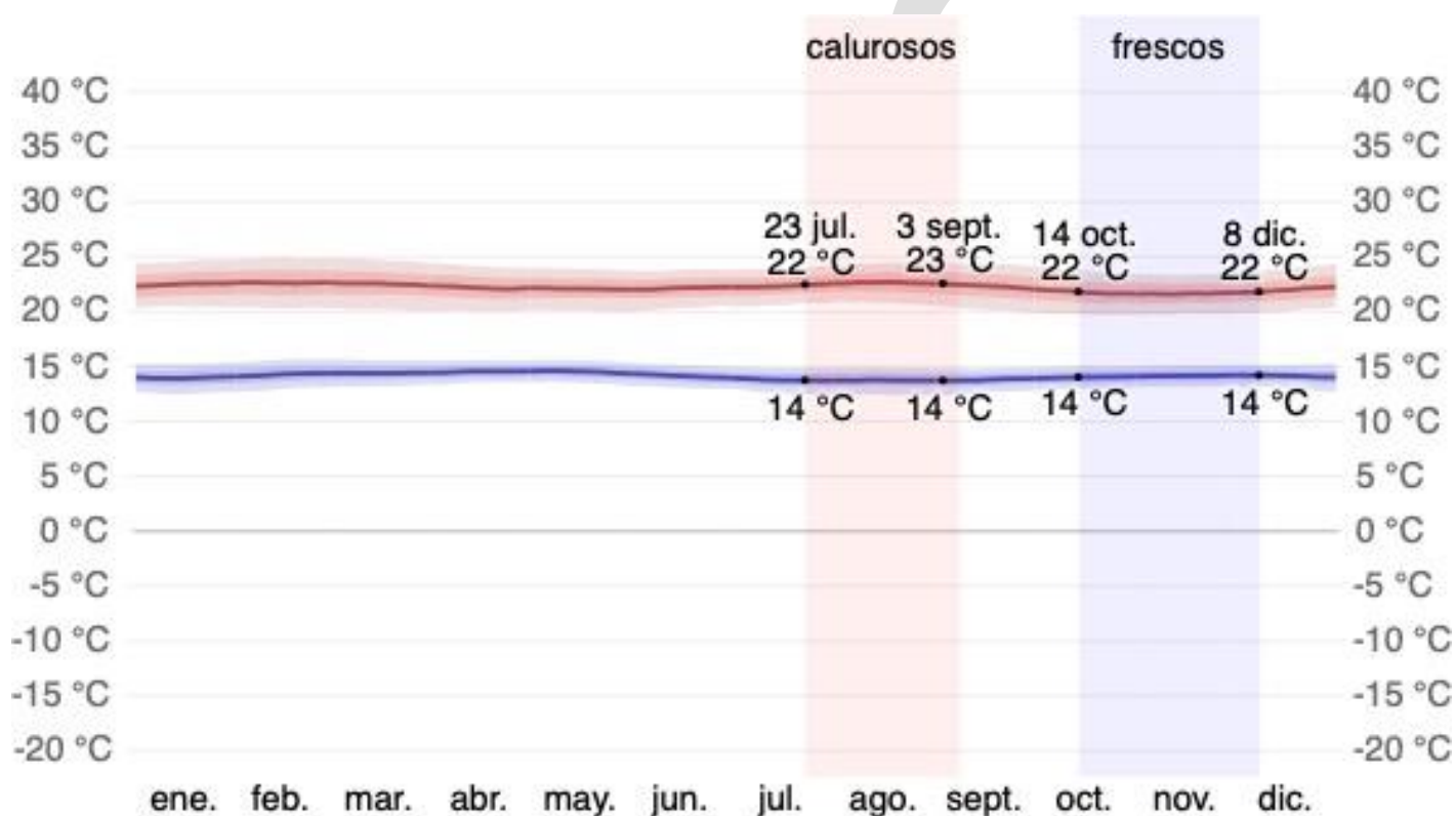
Temperatura máxima y mínima promedio en Manizales
