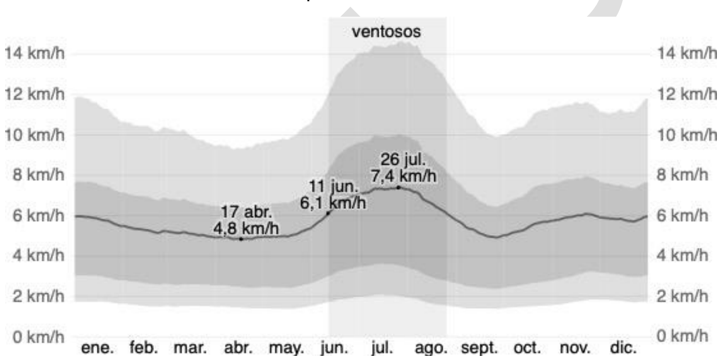
Velocidad promedio del viento en Cali
