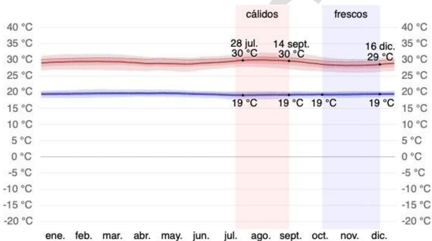
Temperatura máxima y mínima promedio en Cali
