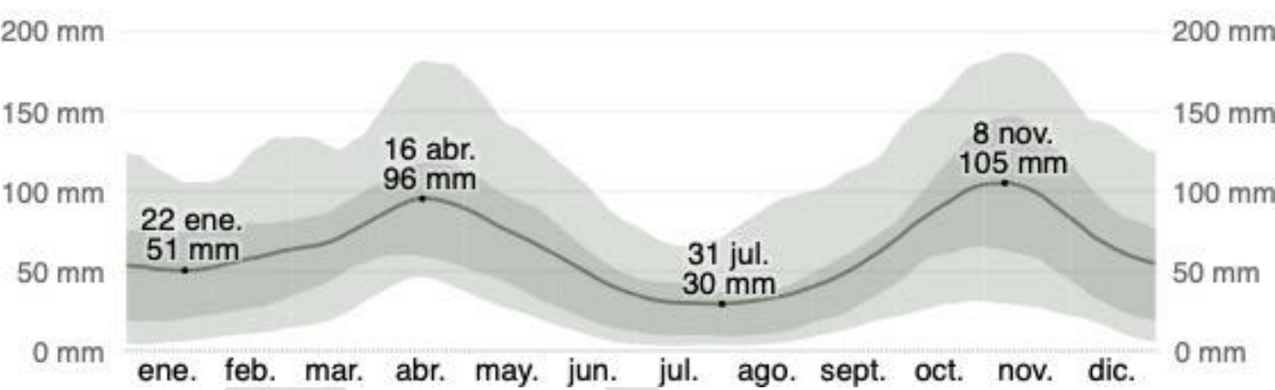
Promedio mensual de lluvia en Cali
